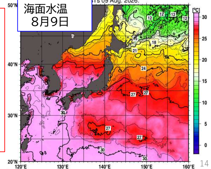
海面水温 Ts 09 Aug. 2026.
